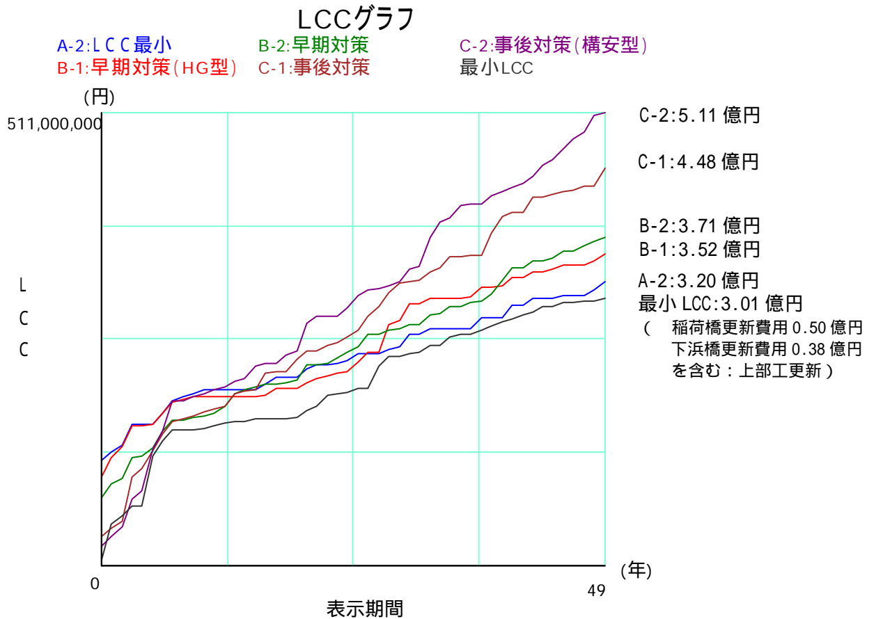
図 5 - 9 シナリオ別LCC算定結果
