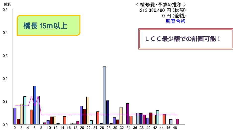
図 5-12 予算制約を考慮した予算シミュレーション結果(橋長 15m 以上)
