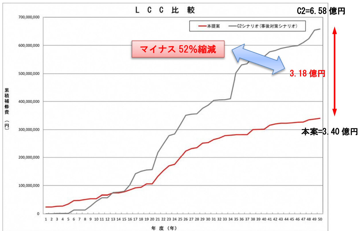
図8-1 橋梁のコスト削減効果
