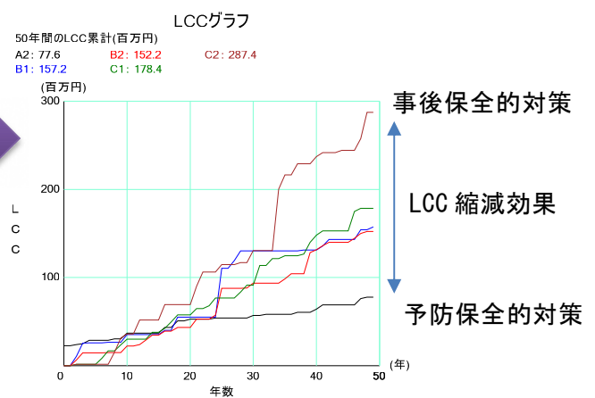
図2 LCCグラフ
