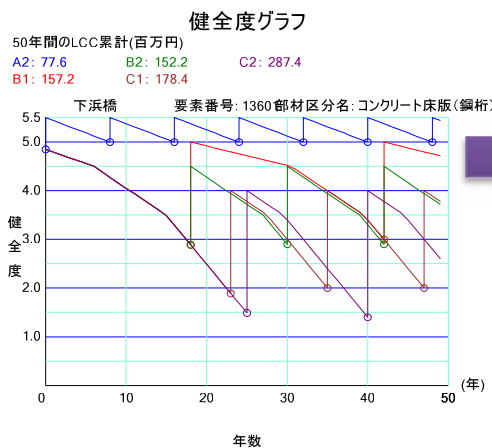
図1 健全度グラフ
