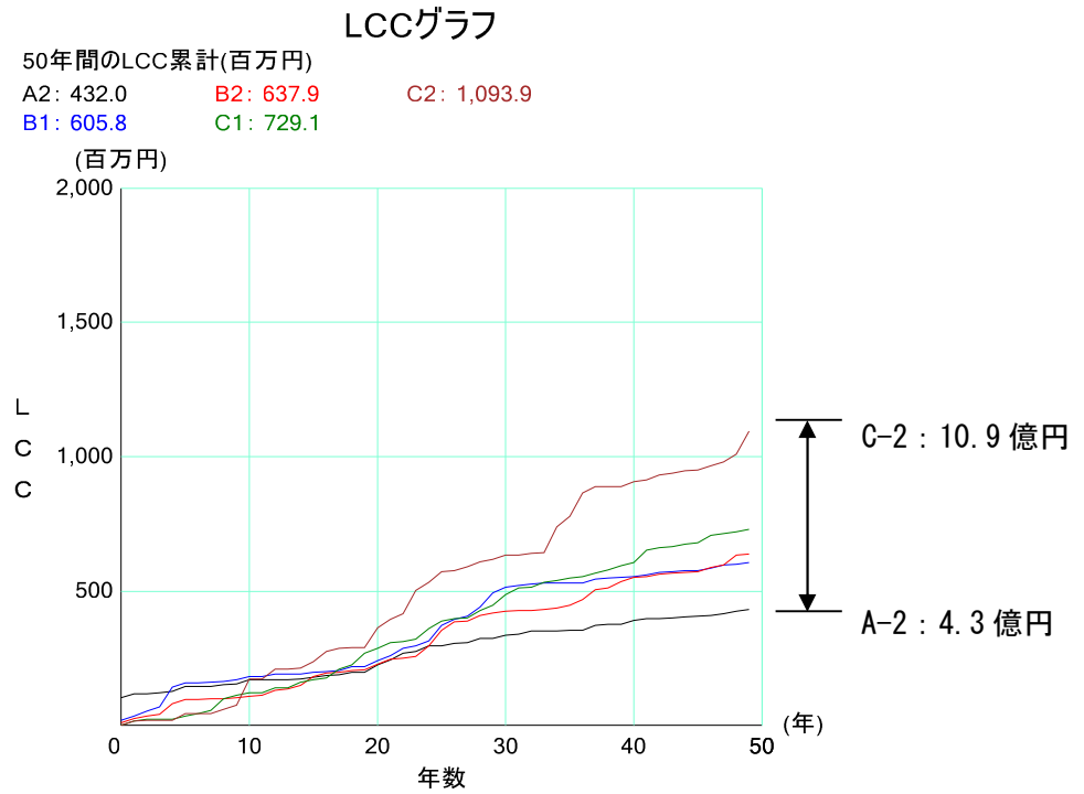
図 7-9 シナリオ別LCC算定結果
