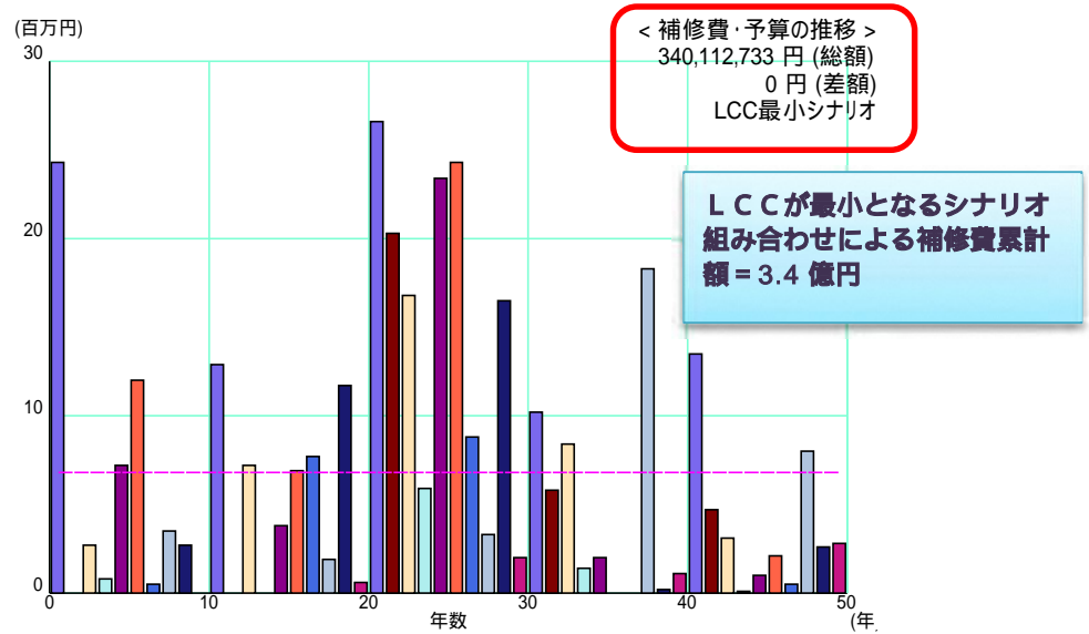
図 7-10 50年間LCCが最小となるシナリオの組み合わせにおける補修費の推移
