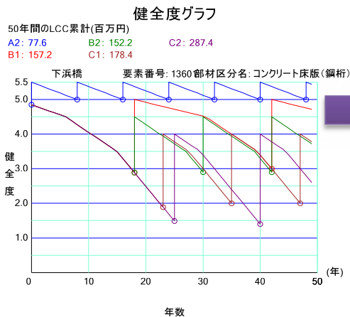
図1 健全度グラフ
