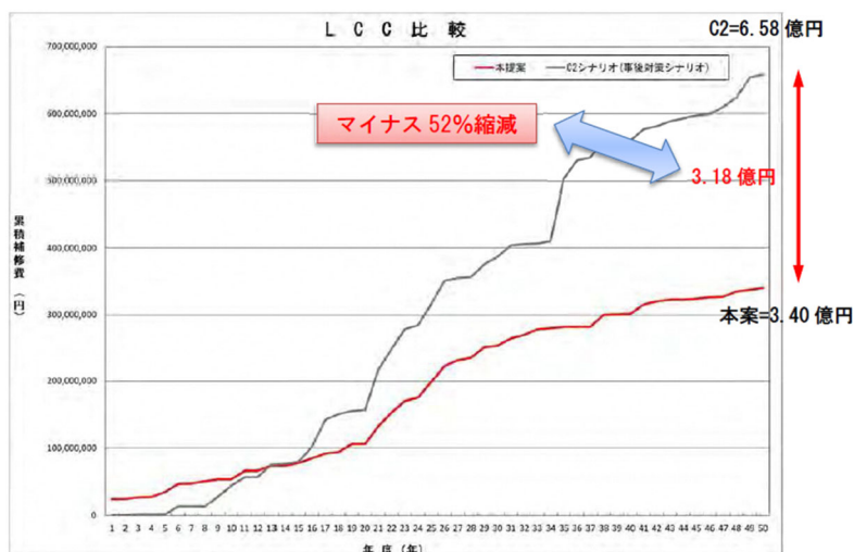
図 8-1 橋梁のコスト縮減効果
